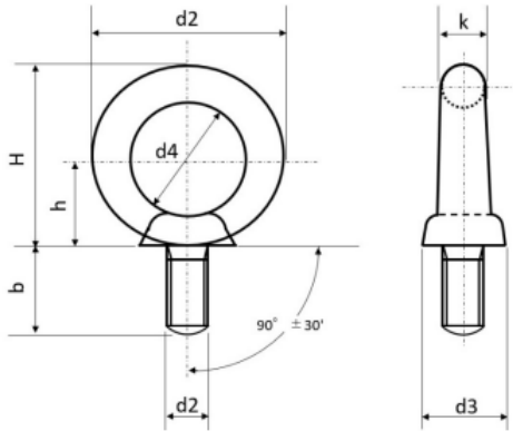
アイボルト JIS B 1168-1994(M 矽)
