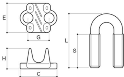
鍛造ワイヤグリップ F型 JIS B2809-1996
